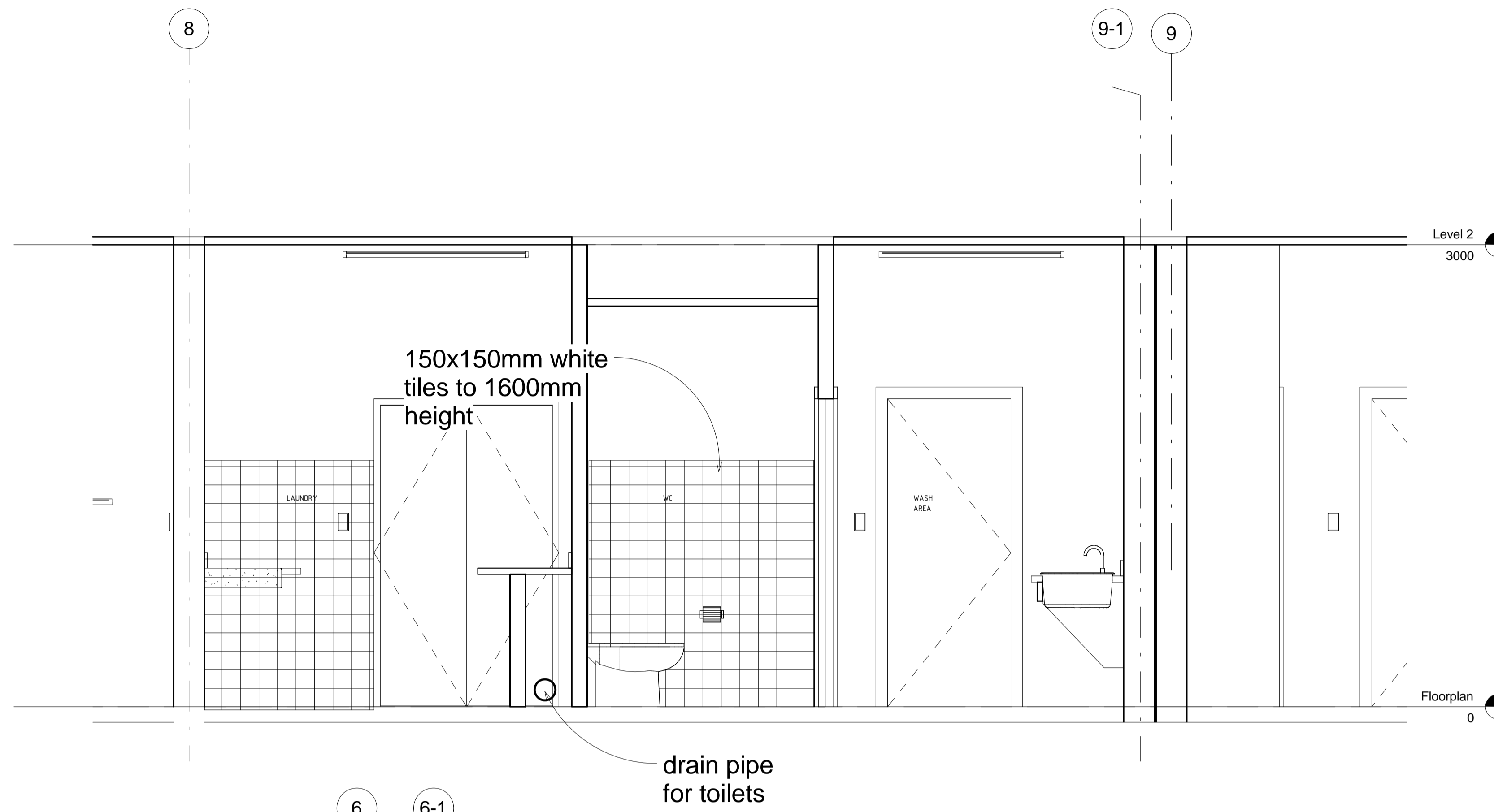
1 Elevation 1 1 : 20
